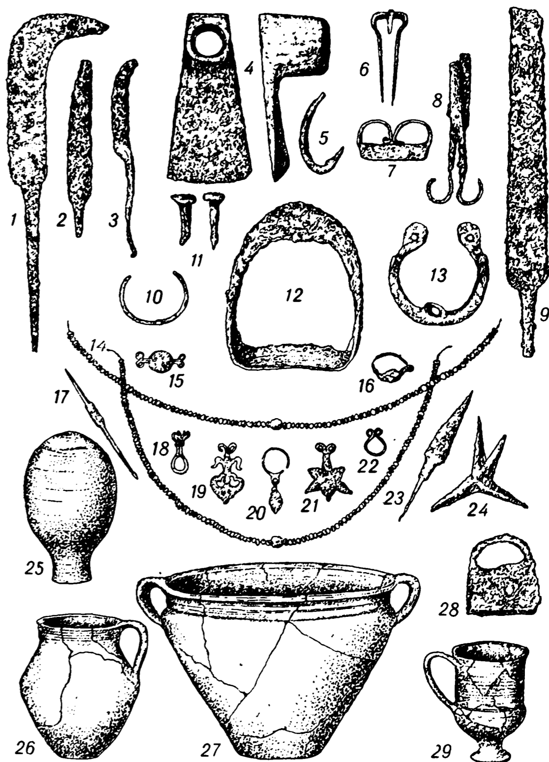
Изделия молдавских ремесленников Старого Орхей 14—16 вв.: 1 — садовый нож; 2 — нож; 3 — закроечный нож; 4 — тесло; 5 — крючок рыболовный; 6 — дрымба (музыкальный инструмент); 7 — кресало; 8 — ножницы; 9 — кинжал; 10 — кабулочная подкова от сапога; 11 — гвозди; 12 — стремя; 13 — подкова; 14 — бусы из разноцветного стекла; 15 — бронзовая застежка с петелькой; 16 — серьга с граненой бусиной; 17 — двухстороннее шило; 18 — петелька от застежки; 19 — золоченая застежка; 20 — золотая серьга с жемчужиной; 21 — золоченая застежка; 22 — бронзовая петелька; 23 — наконечник стрелы; 24 — «чеснок»-шип против неприятельской конницы; 25 — глиняная копилка; 26 и 27 — глиняные сосуды; 28 — замок; 29 — глиняный бокал, покрытый белой глазурью.
